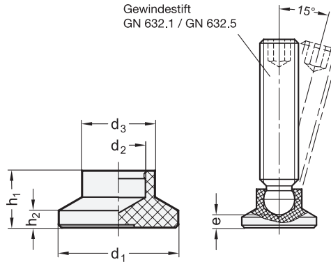
Montagebeispiel
